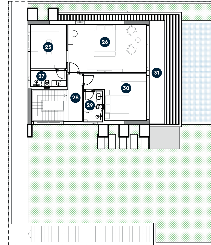
1. Kat Planı
